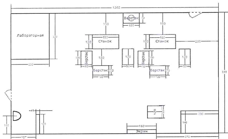
Рисунок 1. Фрезерная мастерская с ЧПУ
