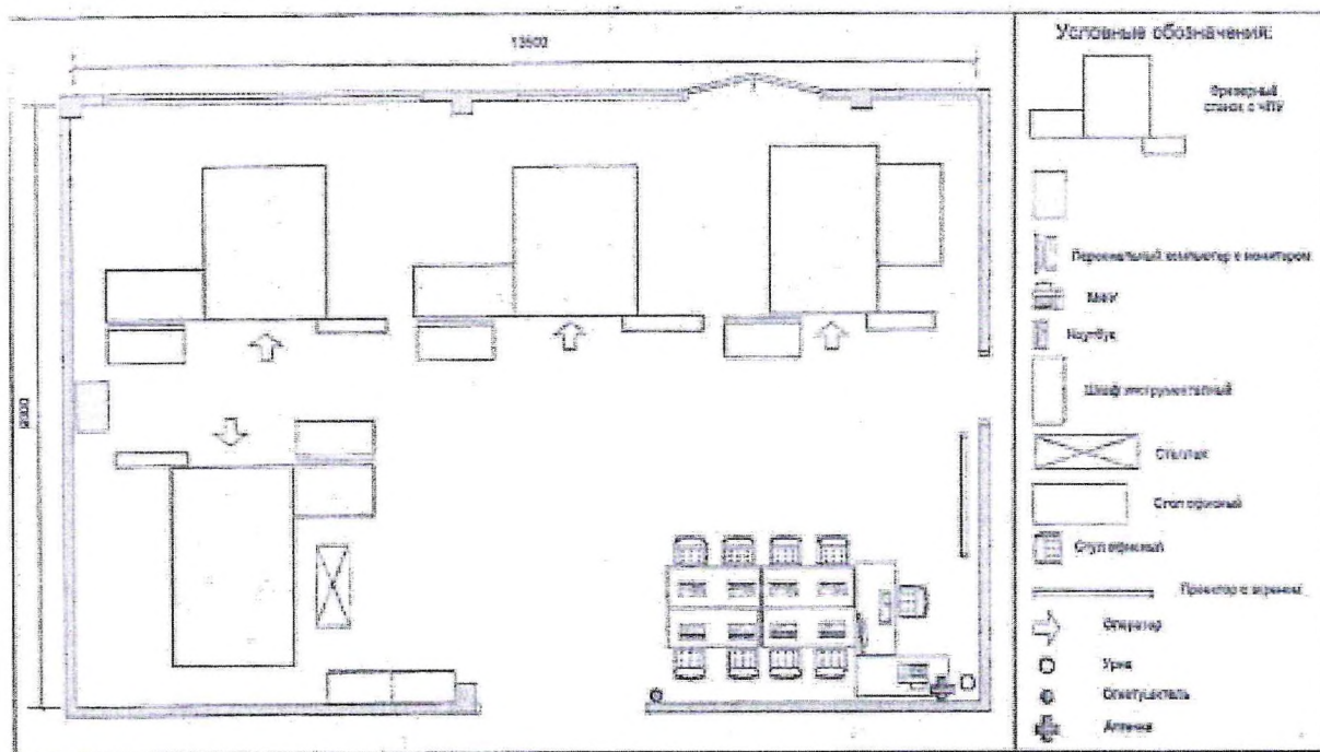
Рисунок 1. Фрезерная мастерская станков с ЧПУ
