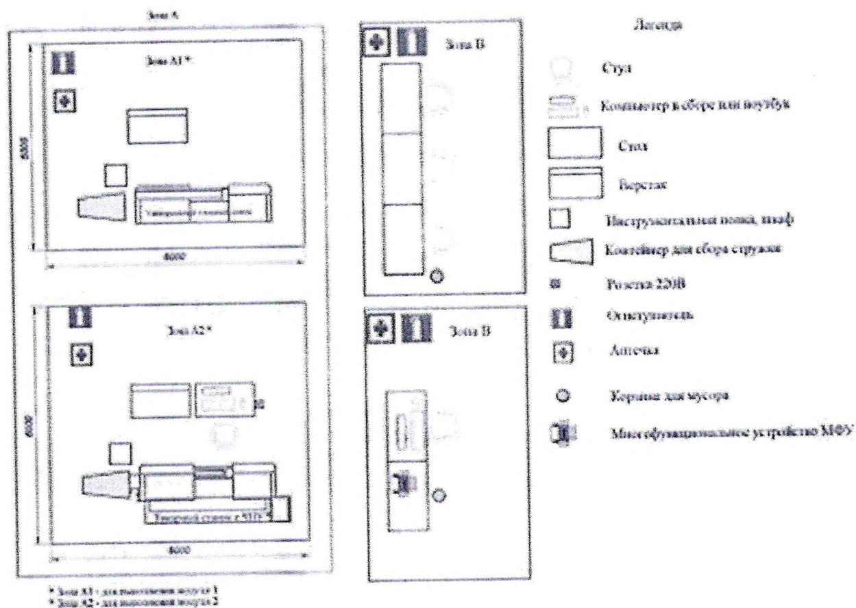
Рисунок 4- Токарная мастерская с ЧПУ.
